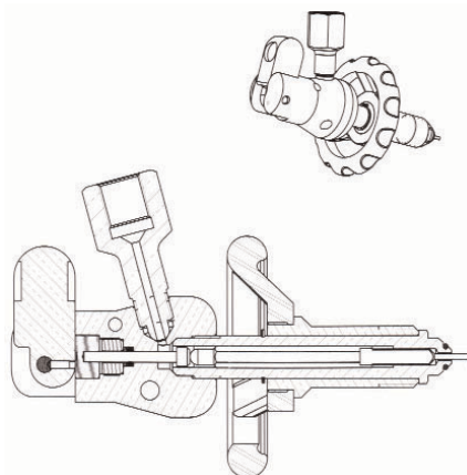
Outil pour robinet à retenue de pression Tool for retained pressure cylinder valve
